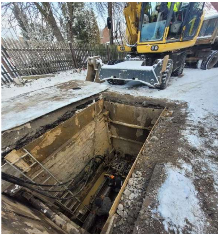
Rysunek 5. Budowa kanalizacji sanitarnej w sołectwie Lubomia wraz z kolektorem przesyłowym do Miasta Racibórz
